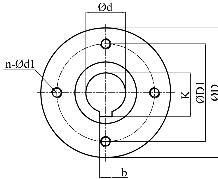
QZ系列气动执行器连接参数表
